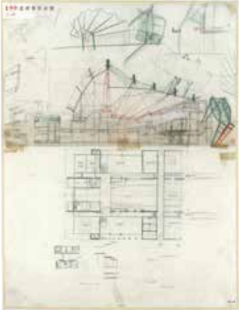
no.120 菊竹清訓 | 都城市民会館 スケッチ | 所蔵：株式会社情報建築 KIKUTAKE Kiyonori | Miyakonojo Civic Center, Sketch | ©KIKUTAKE Kiyonori
